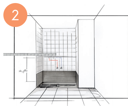
2 Nyní přesuňte přípojky a připravte stěnu
