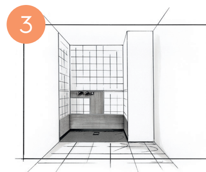
3 Uložte novou vaničku včetně těsnicí pásky
