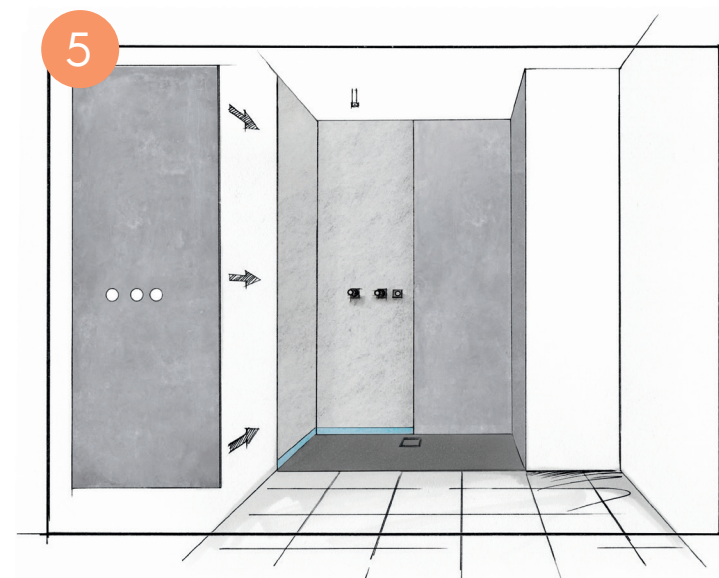
5 Nainstalujte HÜPPE EasyStyle stěnu. Bez nečistot a prachu lze 3mm silné kompozitní hliníkové panely – ve dvou standardních velikostech – řezat a instalovat. Nalepením těsně jedna k druhé bude váš sprchový prostor prakticky beze spár. Případně je možno tyto desky instalovat pomocí úzkých hliníkových profilů
