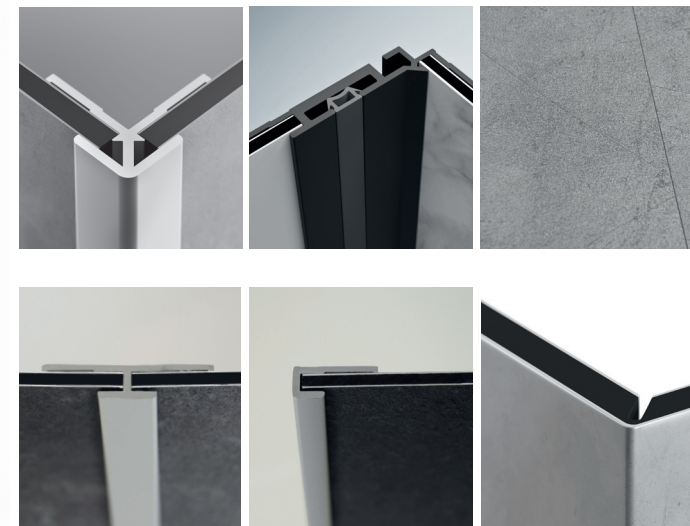
Instalace s hliníkovými profily – K dispozici v 5 vybraných barvách
