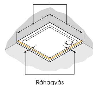
Zuhanytálca beépítési mérete (WEM)
