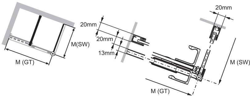
M (SW) a görgőt megvezető sín.
